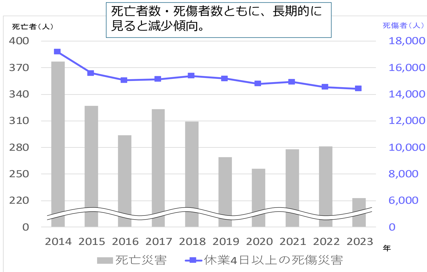
図1-2 死亡者数、休業4日以上之死傷者数推移 (建設業)
