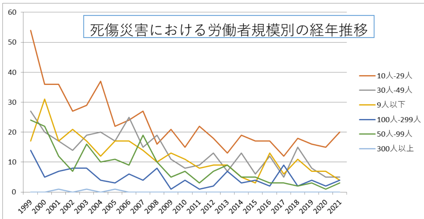
010905 その他の窯業における死傷災害の労働者規模別の経年推移（1999-2021年）
