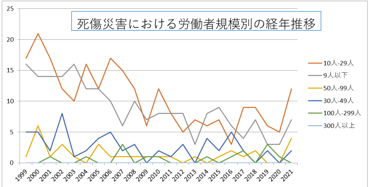
020209その他の土石採取業における死傷災害の労働者規模別の経年推移（1999-2021年）
