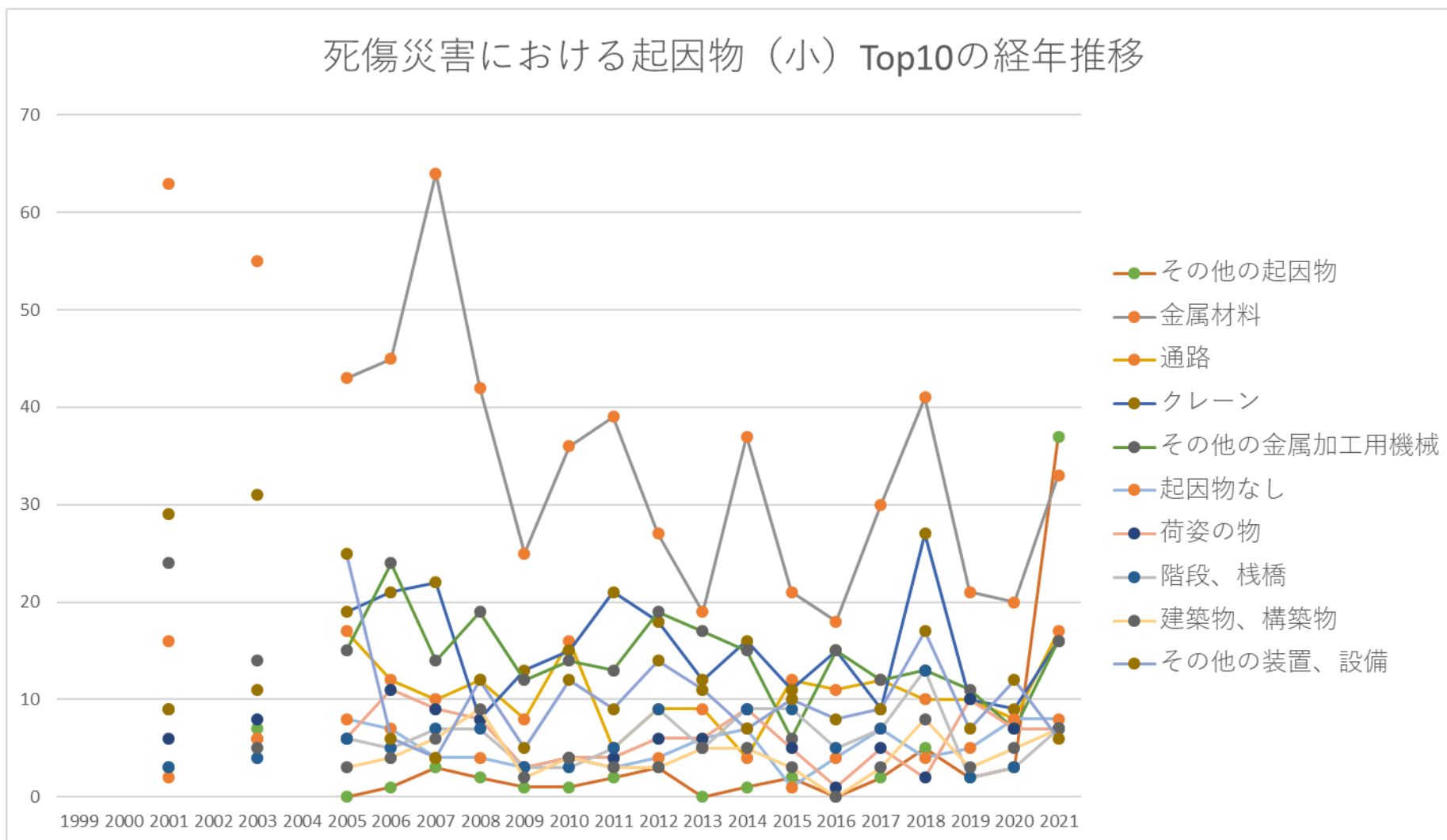
011001製鉄・製鋼・圧延業における死傷災害の事故の型の経年推移（1999-2021年）
