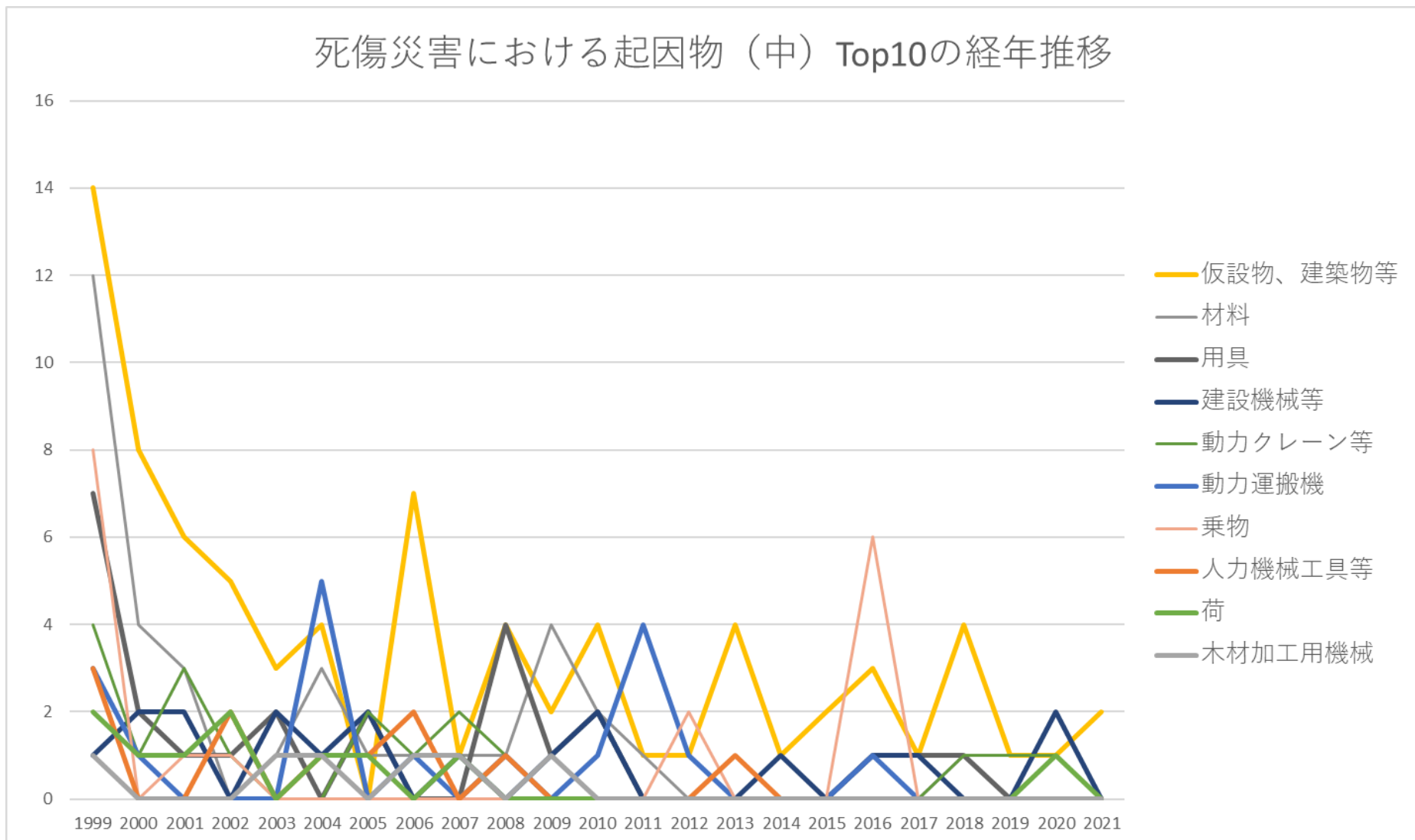
030103地下鉄建設工事における死傷災害の起因物（小）の経年推移（1999-2021年）
