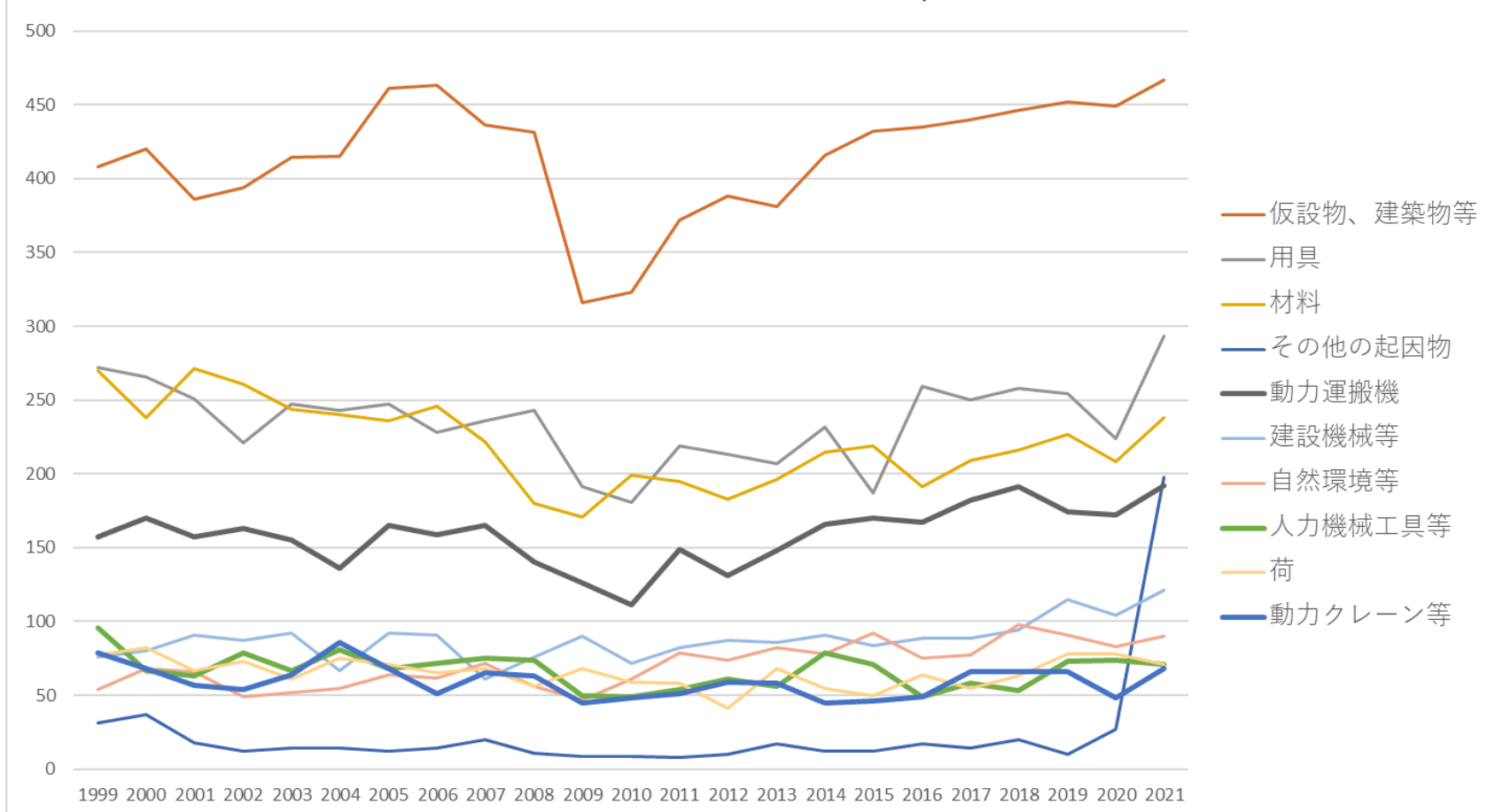
030309その他の建設業－その他における死傷災害の起因物（小）の経年推移（1999-2021年）
