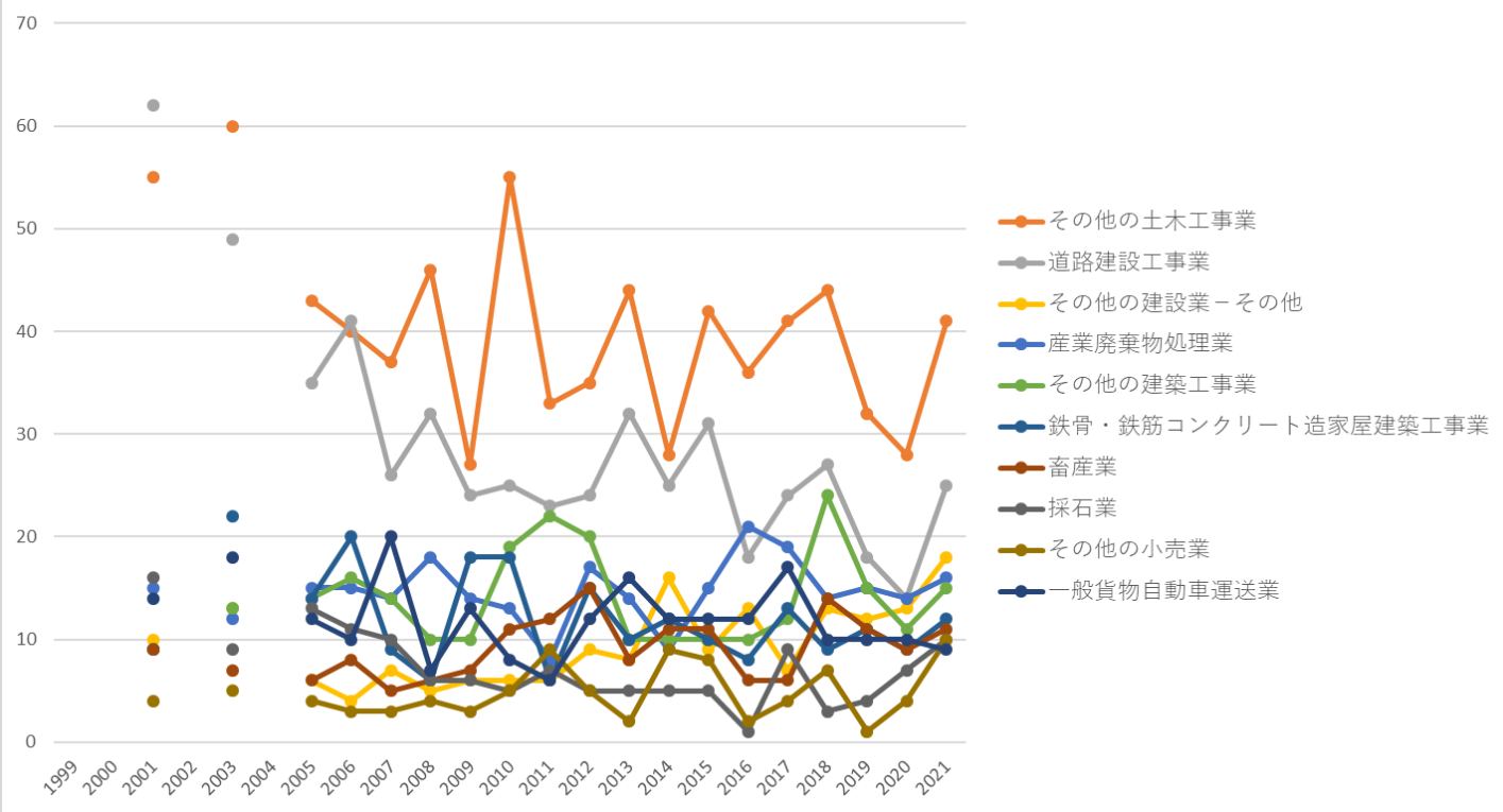
起因物（小）141整地・運搬・積み込み用機械における死傷災害の大業種別の経年推移（1999-2021年）
