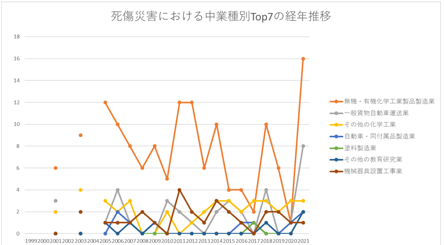
起因物（小）321化学設備における死傷災害の中業種別Top7の経年推移（1999-2021年）
