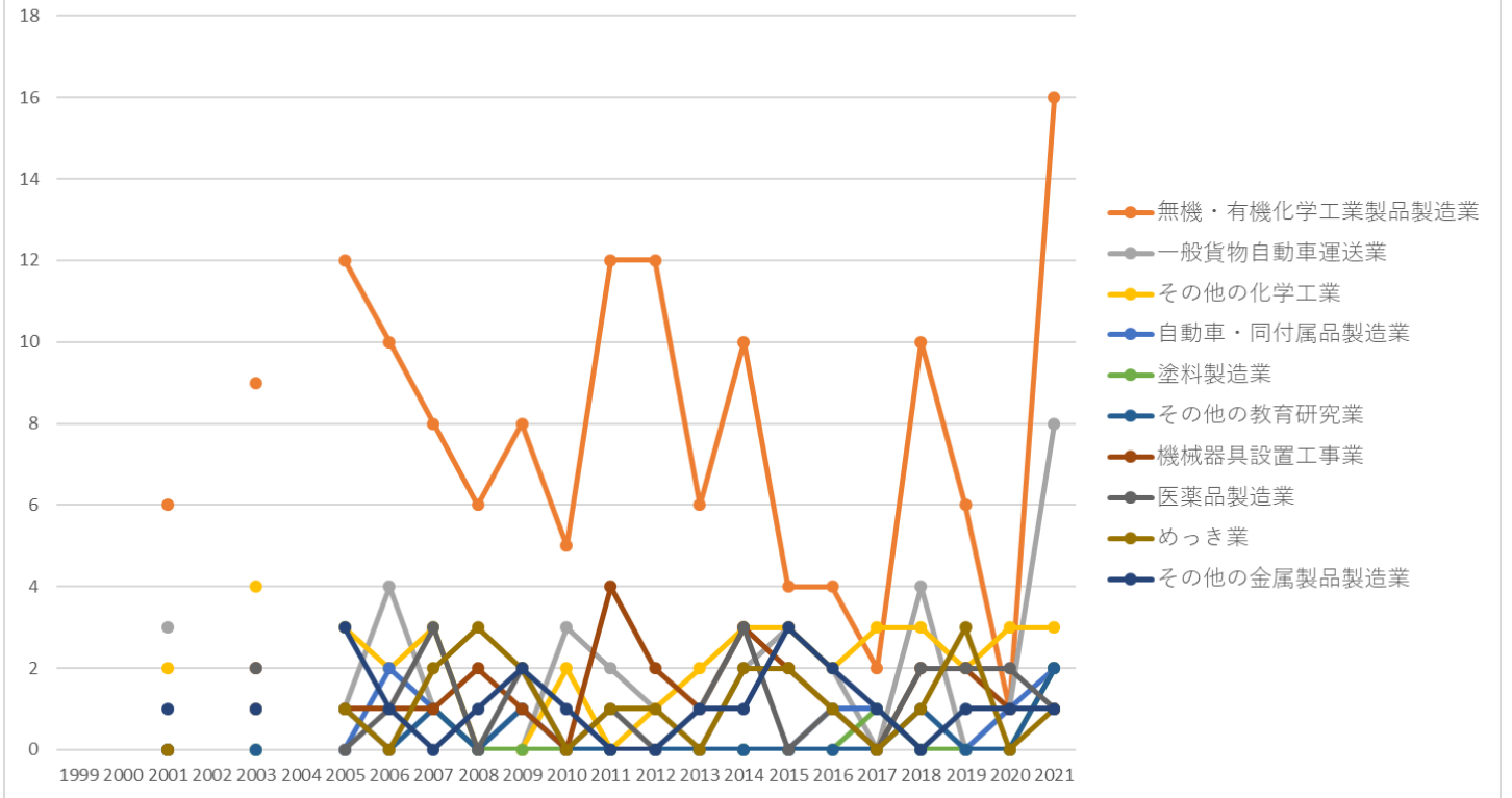
起因物 (小) 321化学設備における死傷災害の大業種別の経年推移 (1999-2021年)
