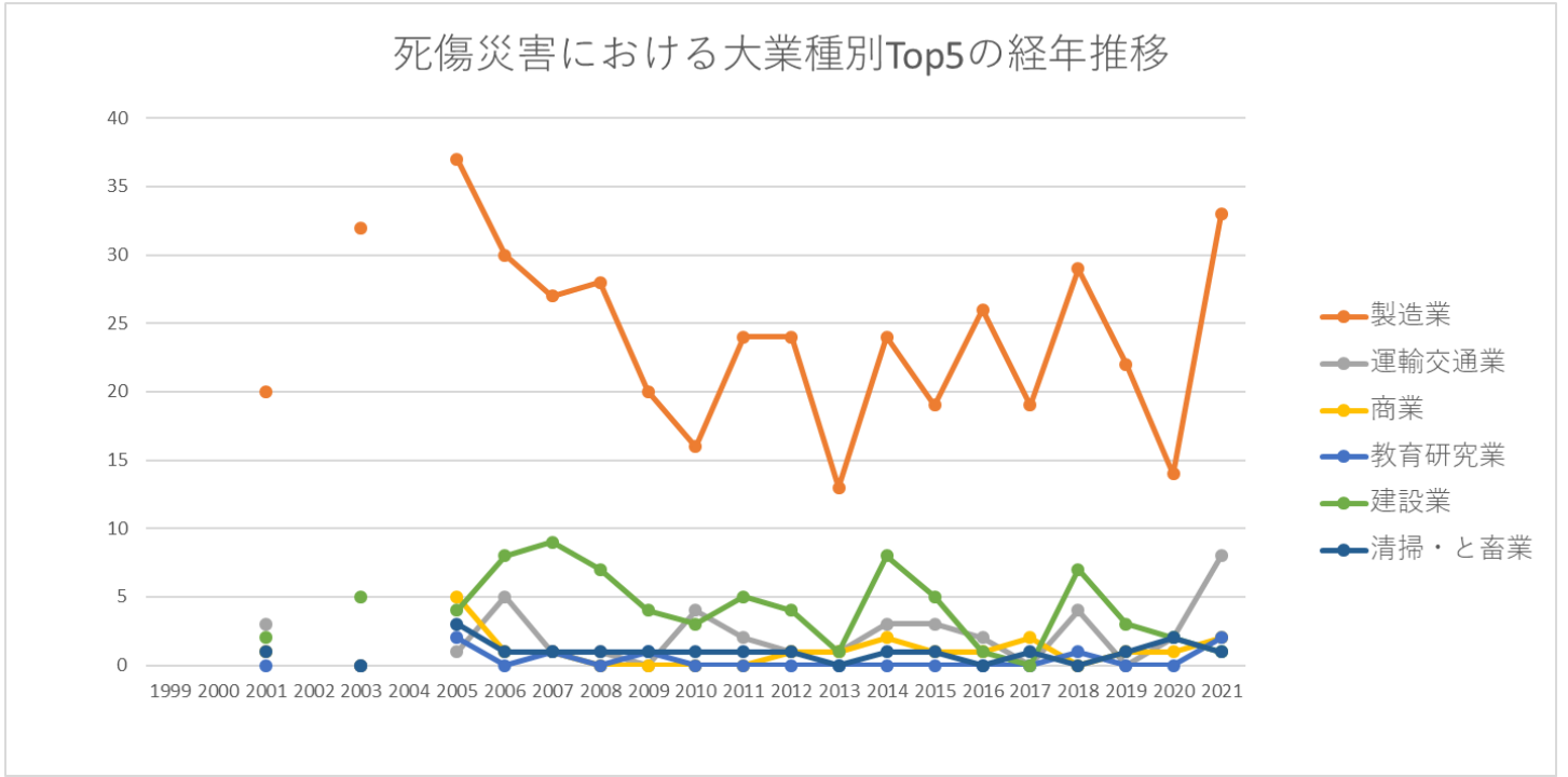
起因物（小）321化学設備における死傷災害の大業種別Top5の経年推移（1999-2021年）
