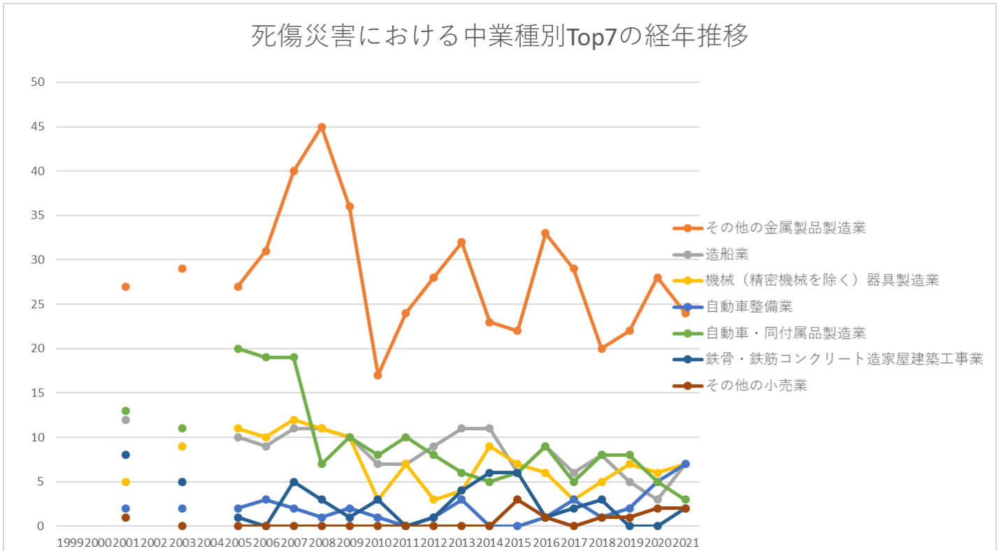
起因物 (小) 332アーク溶接装置における死傷災害の中業種別Top7の経年推移 (1999-2021年)
