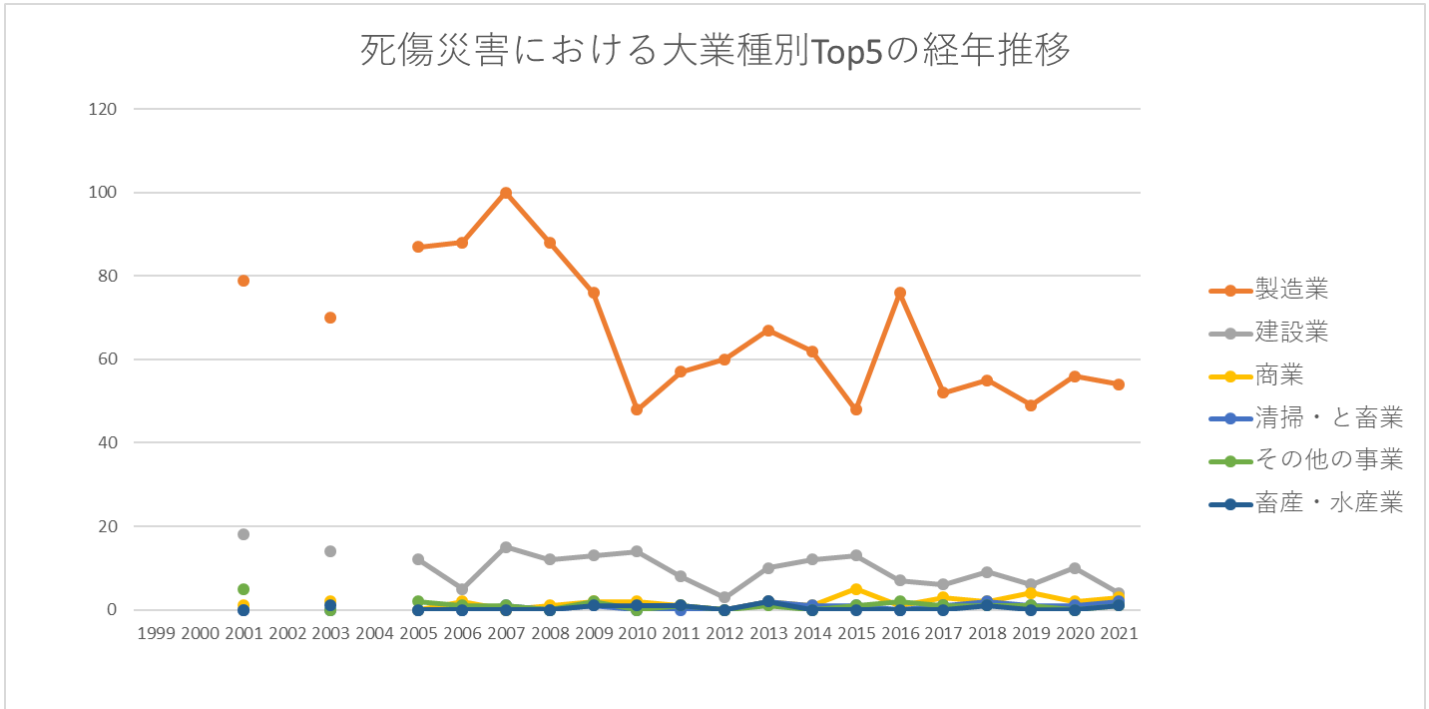
起因物 (小) 332アーク溶接装置における死傷災害の大業種別Top5の経年推移 (1999-2021年)
