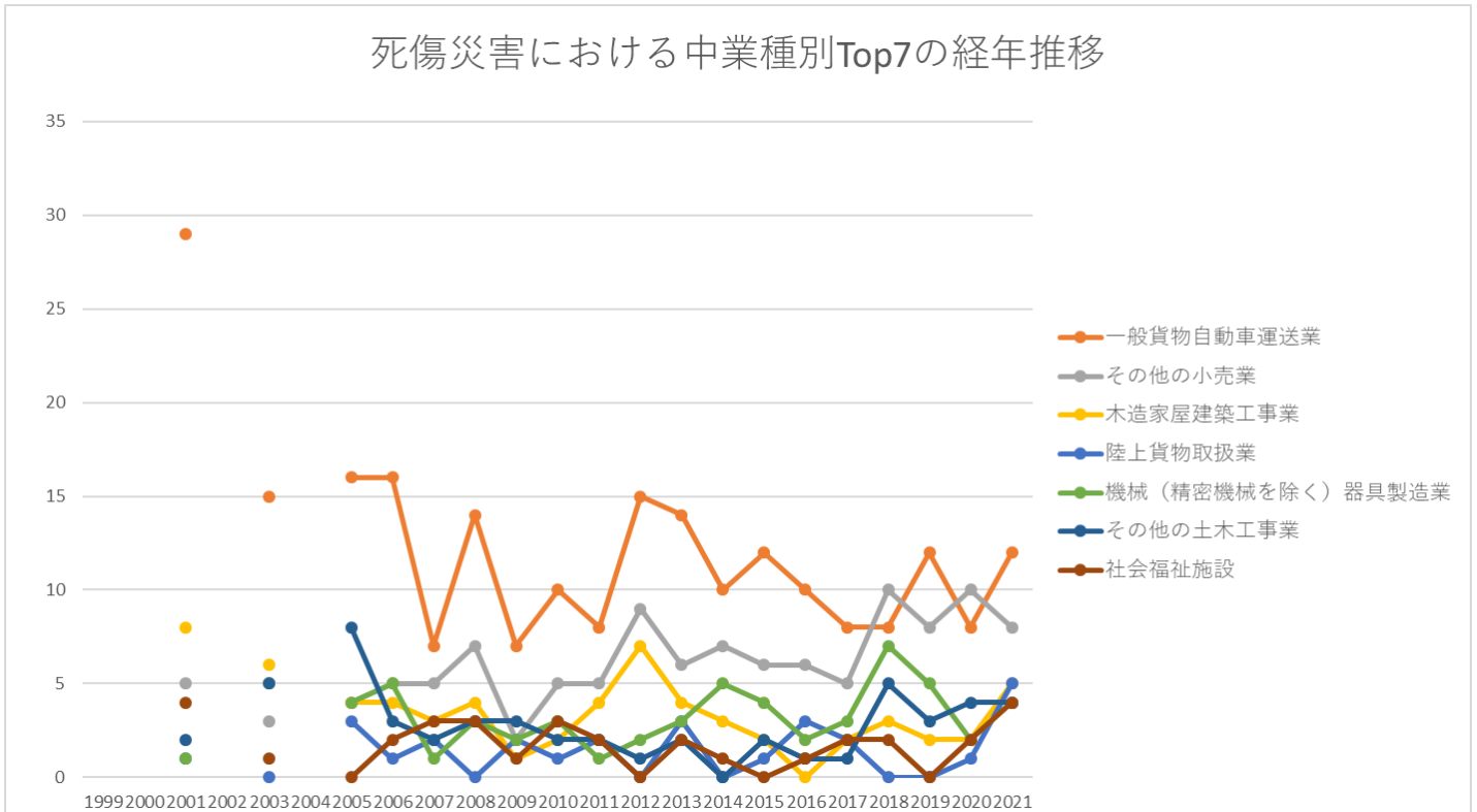
起因物（小）363人力機械における死傷災害の中業種別Top7の経年推移（1999-2021年）
