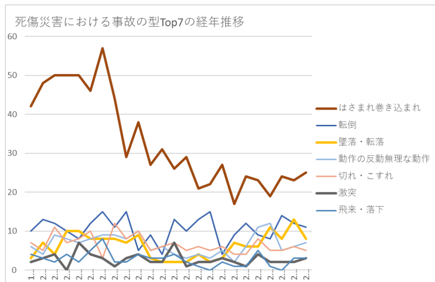
010709 その他の印刷・製本業における死傷災害の事故の型の経年推移（1999-2022年）
