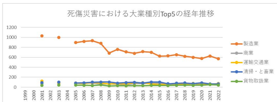
起因物（小） 224 コンベアにおける死傷災害の大業種別Top5の経年推移（1999-2022年）
