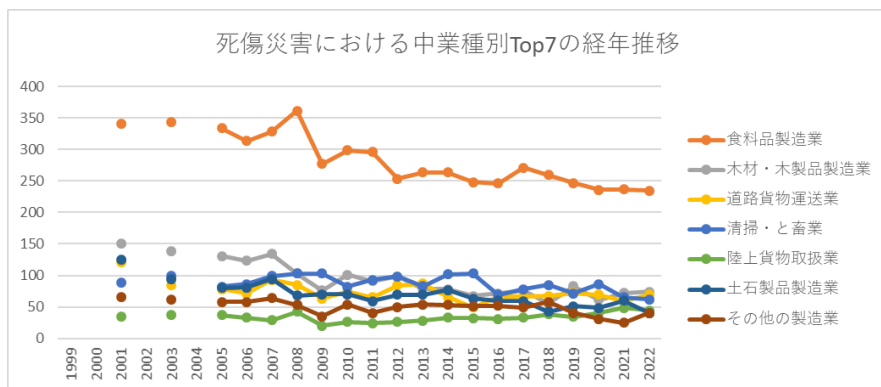
起因物（小） 224 コンベアにおける死傷災害の中業種別Top7の経年推移（1999-2022年）
