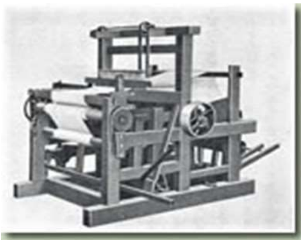
豊田式木鉄混製動力織機
